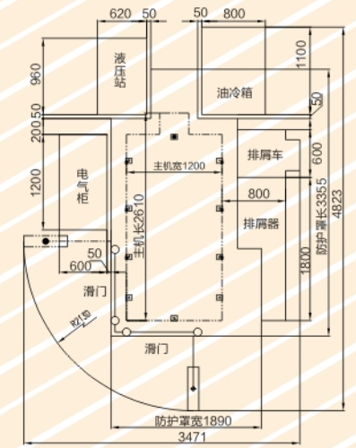
YK8532机床平面布局图
