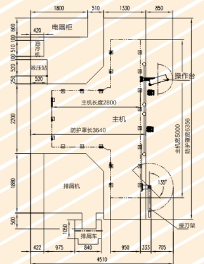
YK85200机床平面布局图
